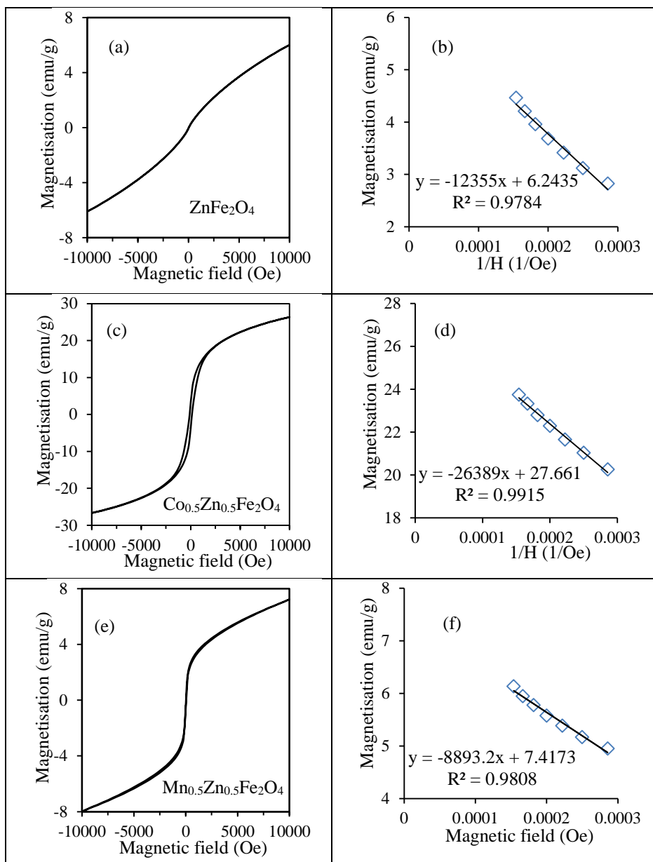
شکل ۶: (a, c, e) منحنی هیستریزیس نمونه‌های ZnFe 2 O 4 , Co 0.5 Zn 0.5 Fe 2 O 4 و Mn 0.5 Zn 0.5 Fe 2 O 4 و (b, d, f) نمودار مغناطش بر حسب عکس میدان در میدان‌های اعمالی بزرگ.
