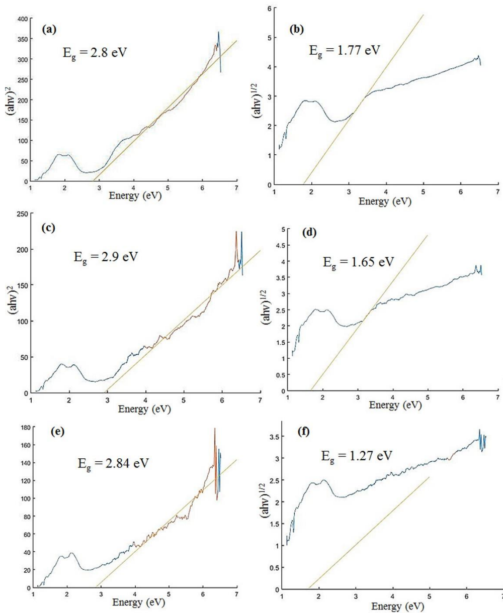
شکل ۵: (a) تخمین گاف انرژی غیرمستقیم نانوذرات ZnFe 2 O 4 , (b) تخمین گاف انرژی مستقیم نانوذرات ZnFe 2 O 4 , (c) تخمین گاف انرژی غیرمستقیم نانوذرات Co 0.5 Zn 0.5 Fe 2 O 4 , (d) تخمین گاف انرژی مستقیم نانوذرات Co 0.5 Zn 0.5 Fe 2 O 4 , (e) تخمین گاف انرژی غیرمستقیم نانوذرات Mn 0.5 Zn 0.5 Fe 2 O 4 و (f) تخمین گاف انرژی مستقیم نانوذرات Mn 0.5 Zn 0.5 Fe 2 O 4 .
